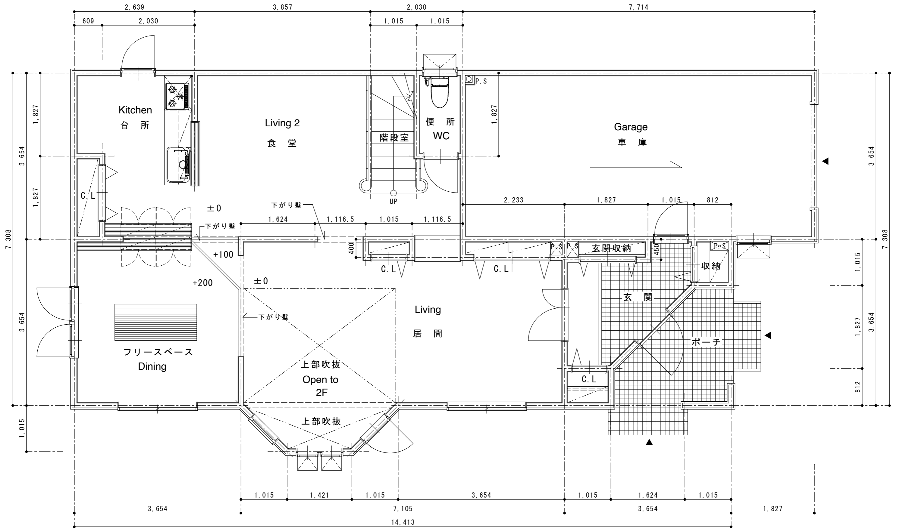
1 F 平面図
